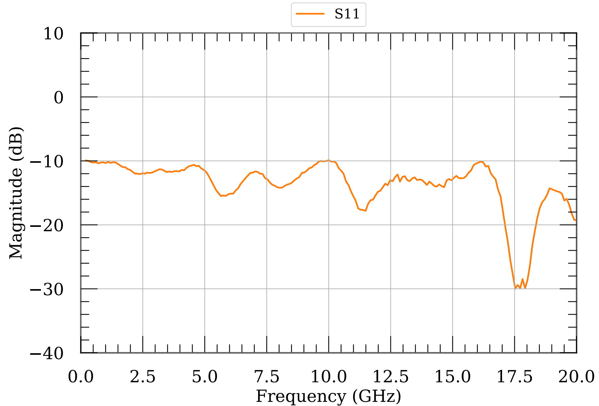
LNA S-params module004v2
